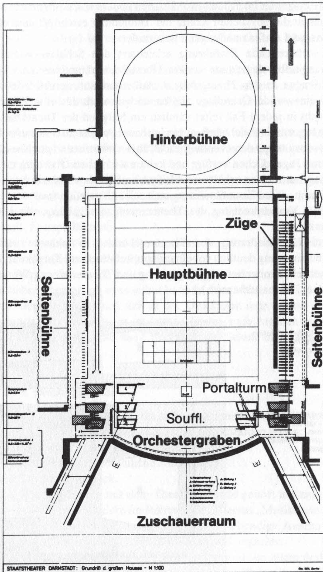
Abb. 14: Grundriß eines modernen Opernhauses (Staatstheater Darmstadt, Großes Haus)
